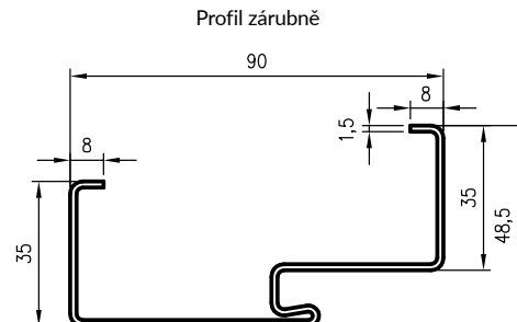
Profil zárubně
